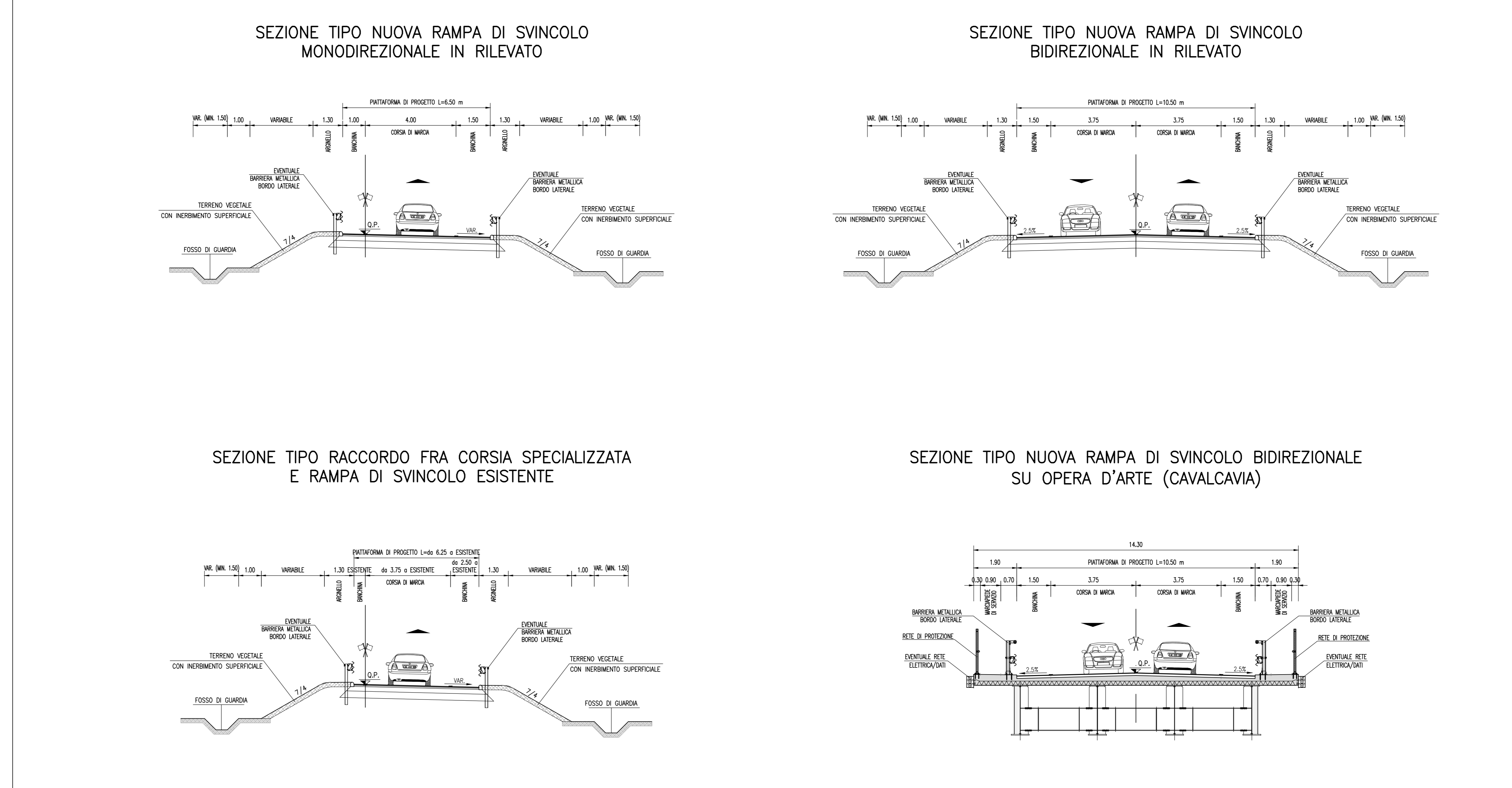
SEZIONE TIPO scala 1:100
