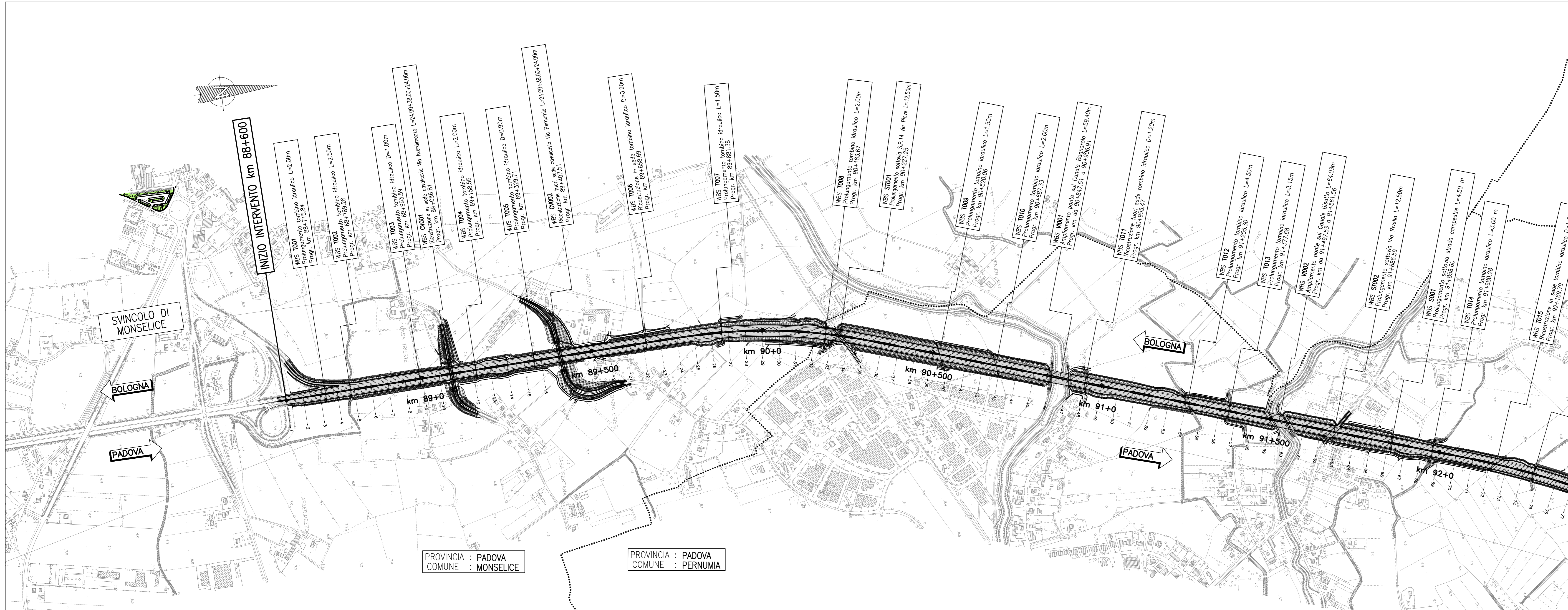
QUADRO 1 - PLANIMETRIA DI PROGETTO dal km 88+600 al km 91+500 - 1:5.000
