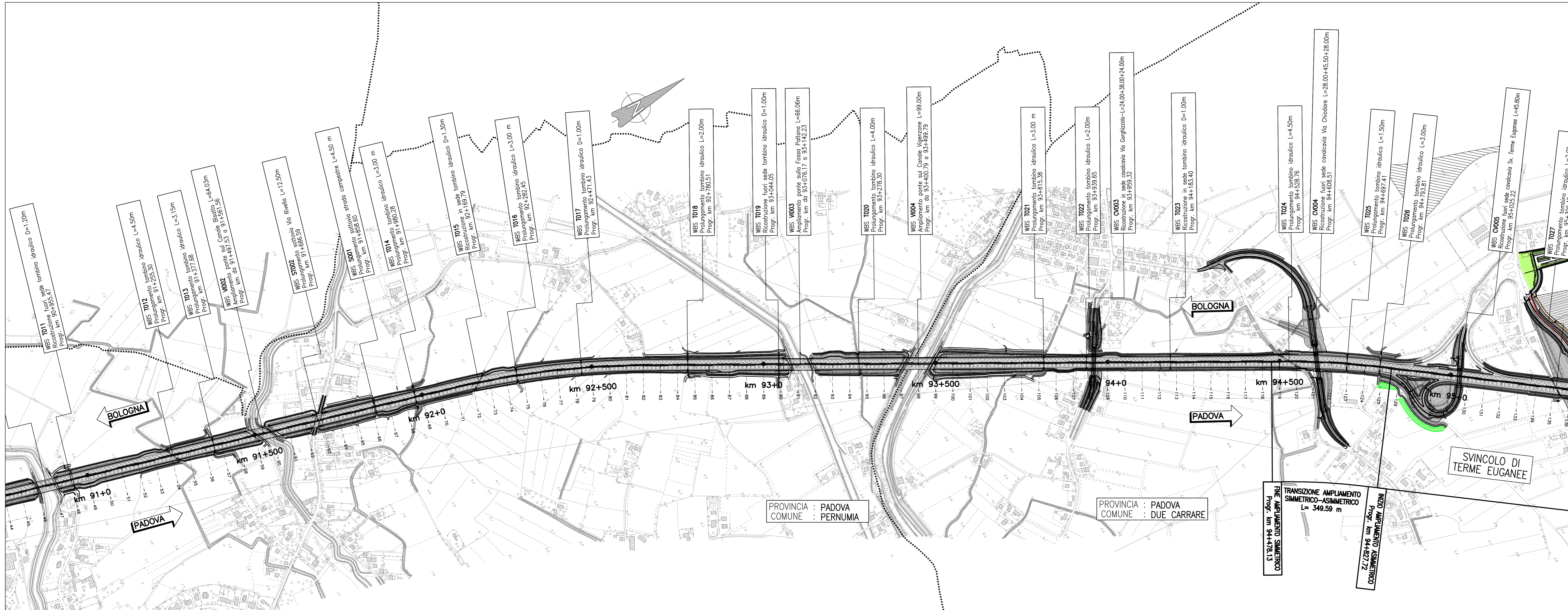
QUADRO 2 - PLANIMETRIA DI PROGETTO dal km 91+500 al km 94+500 - 1:5.000
