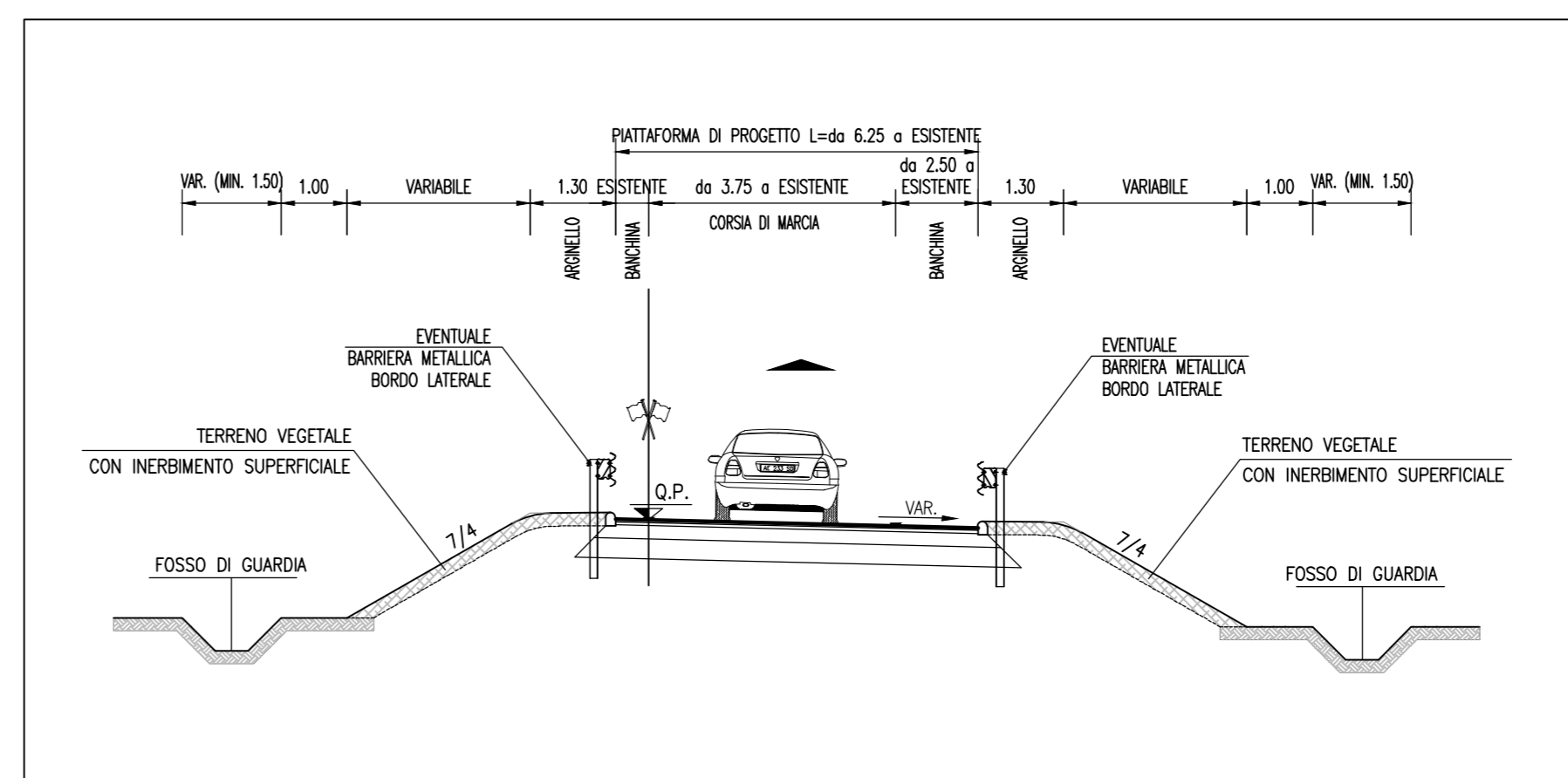
SEZIONE TIPO scala 1:100
