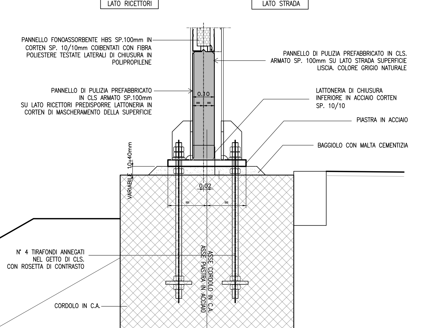
SEZIONE TRASVERSALE 1:50
