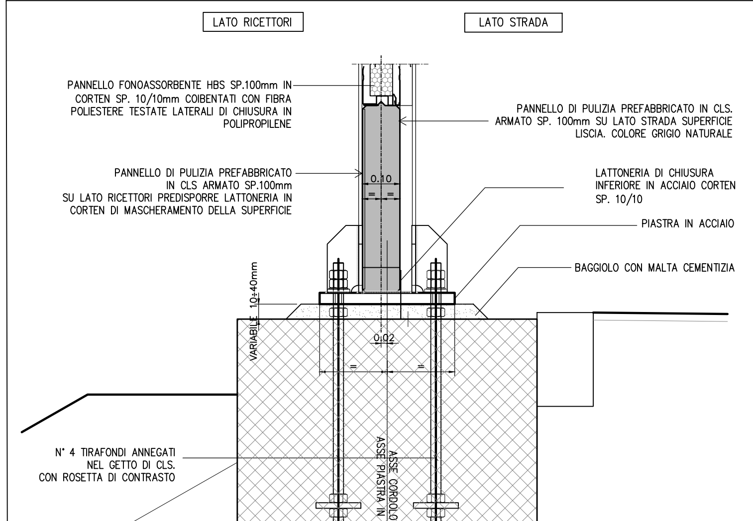
DETTAGLIO 1 1:10
