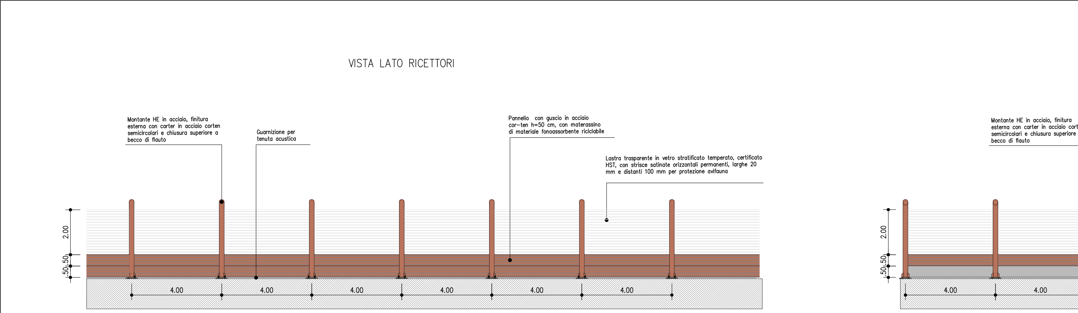
DETTAGLIO "A" - Barriera tipo 1A H3 - Trasparente 1:100
