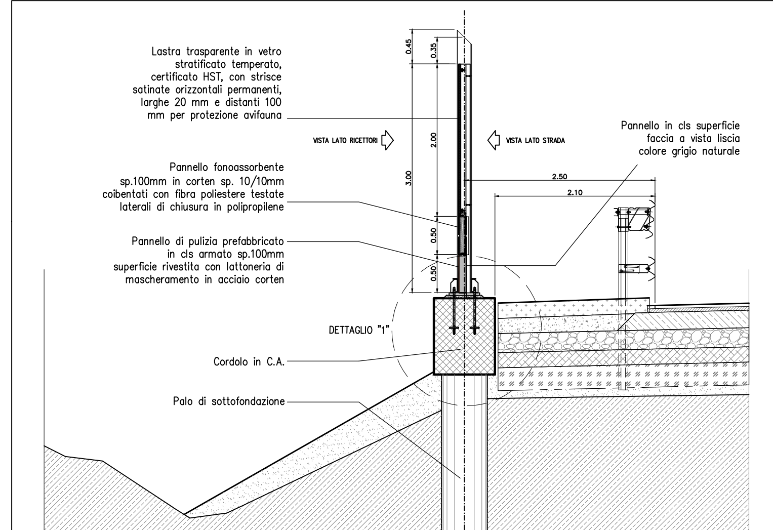
SEZIONE TRASVERSALE 1:50
