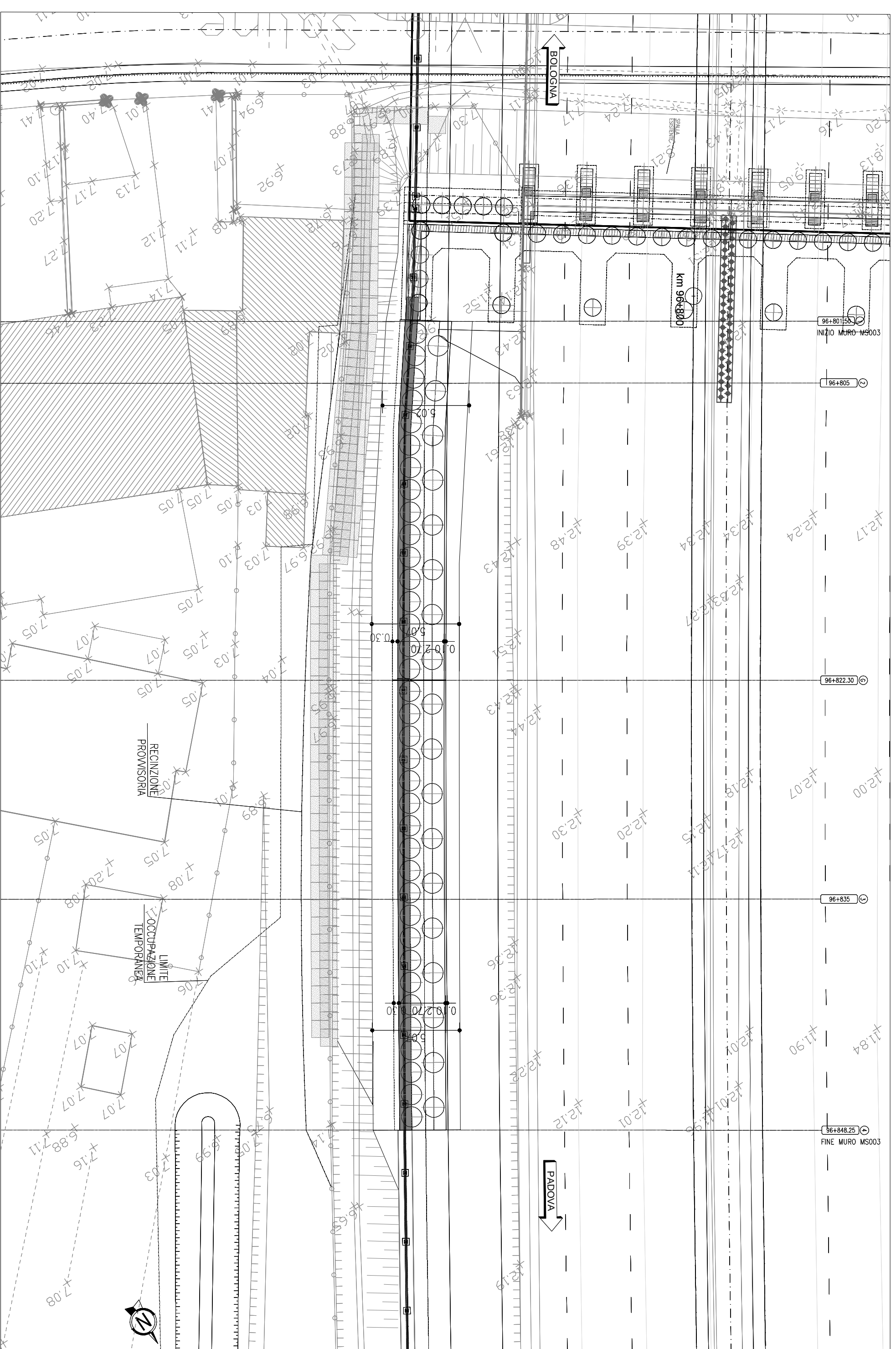
PIANTA-FONDAZIONI (Configurazione in fase di scavo) 1.200
