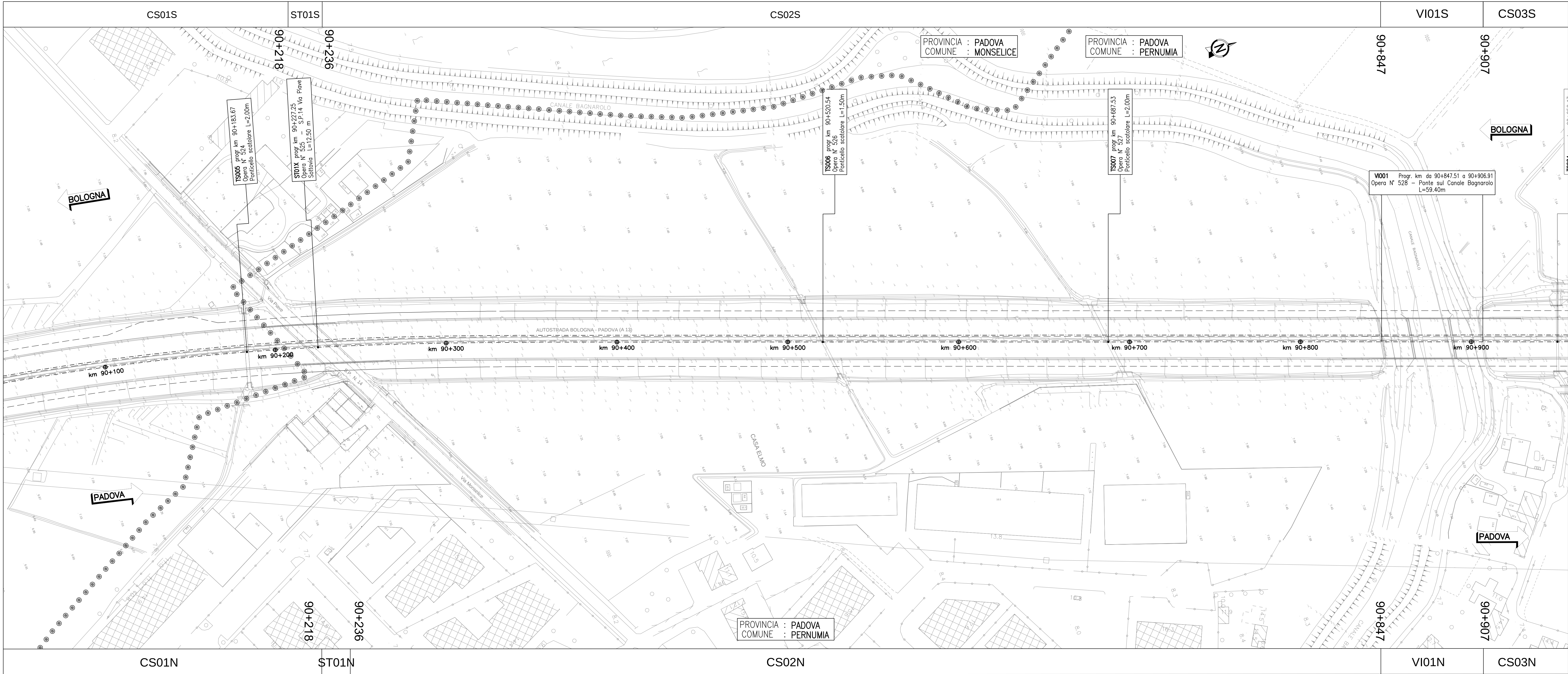
QUADRO 4 – PLANIMETRIA STATO DI FATTO dal km 90+900 al km 91+700 – 1:1.000
