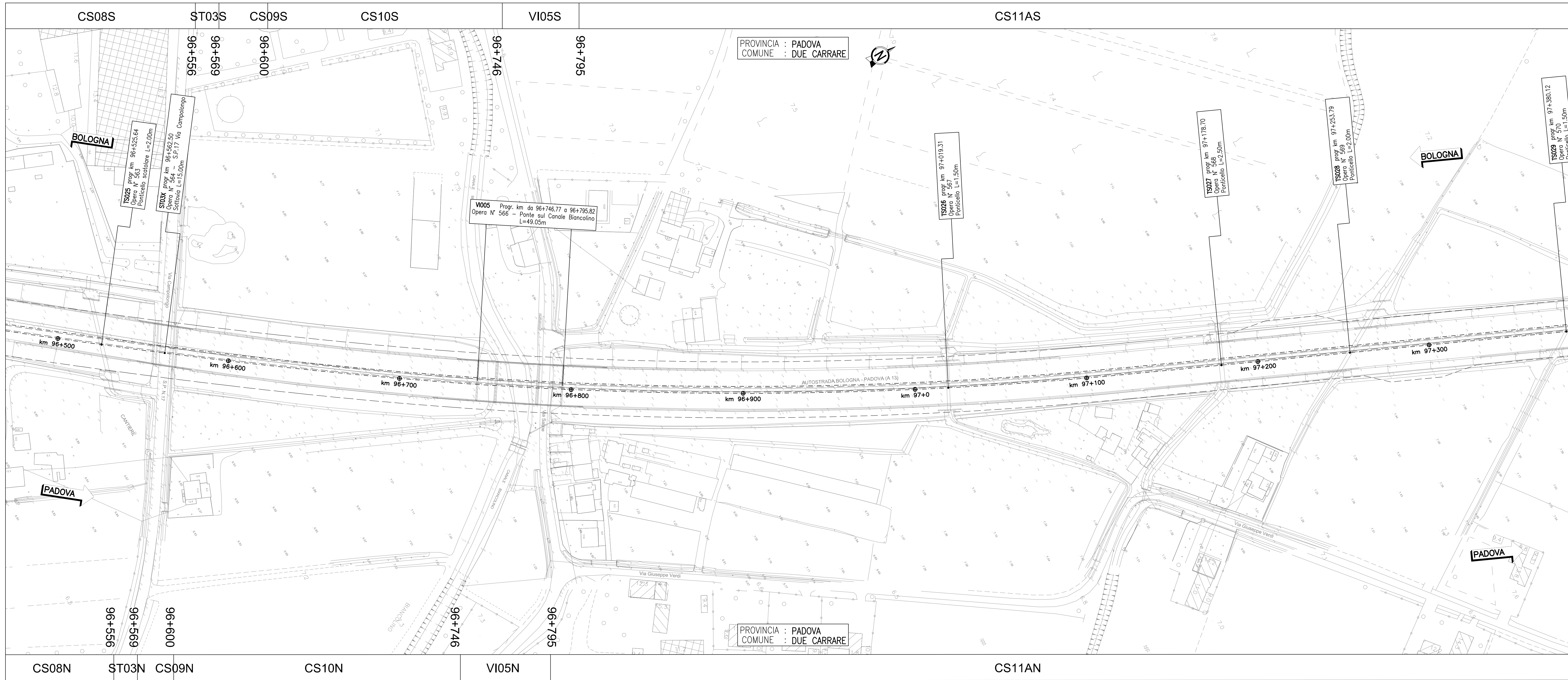
QUADRO 12 – PLANIMETRIA STATO DI FATTO dal km 97+300 al km 98+100 – 1:1.000
