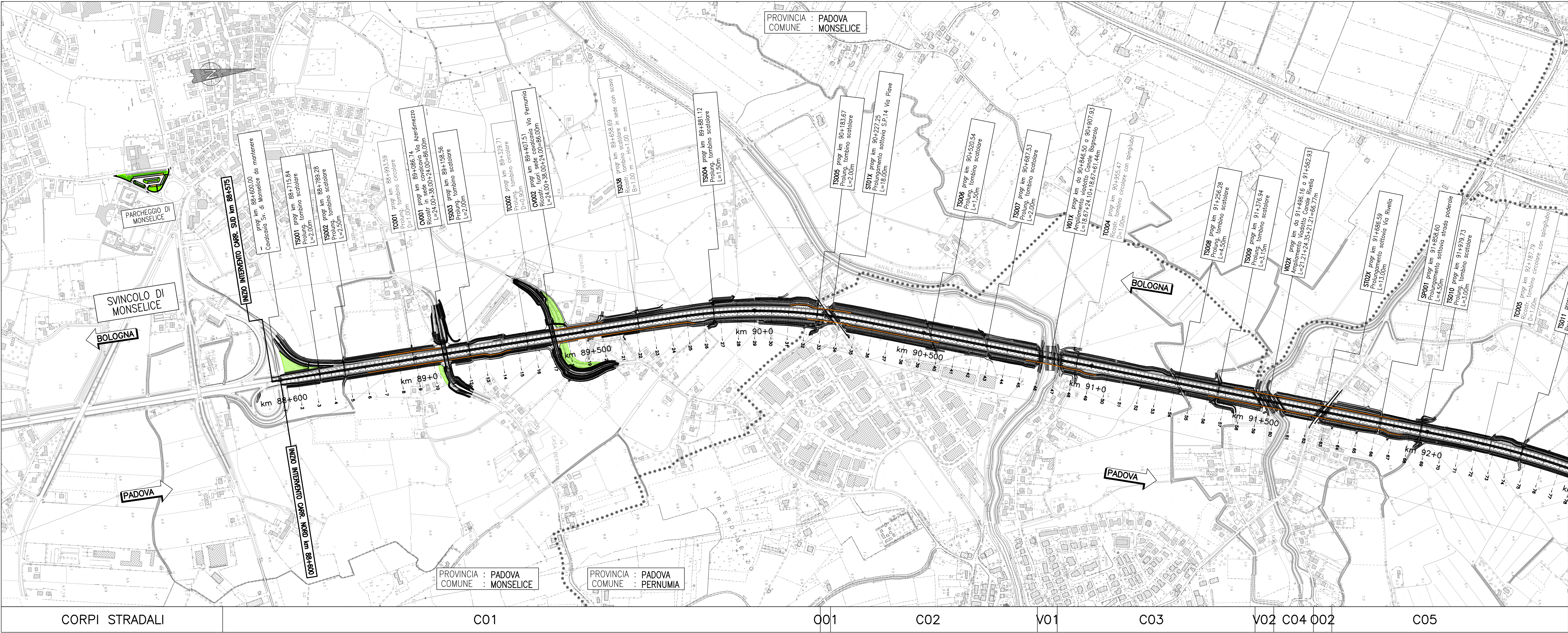
QUADRO 1 – PLANIMETRIA DI PROGETTO dal km 88+575 al km 91+500 – 1:5.000
