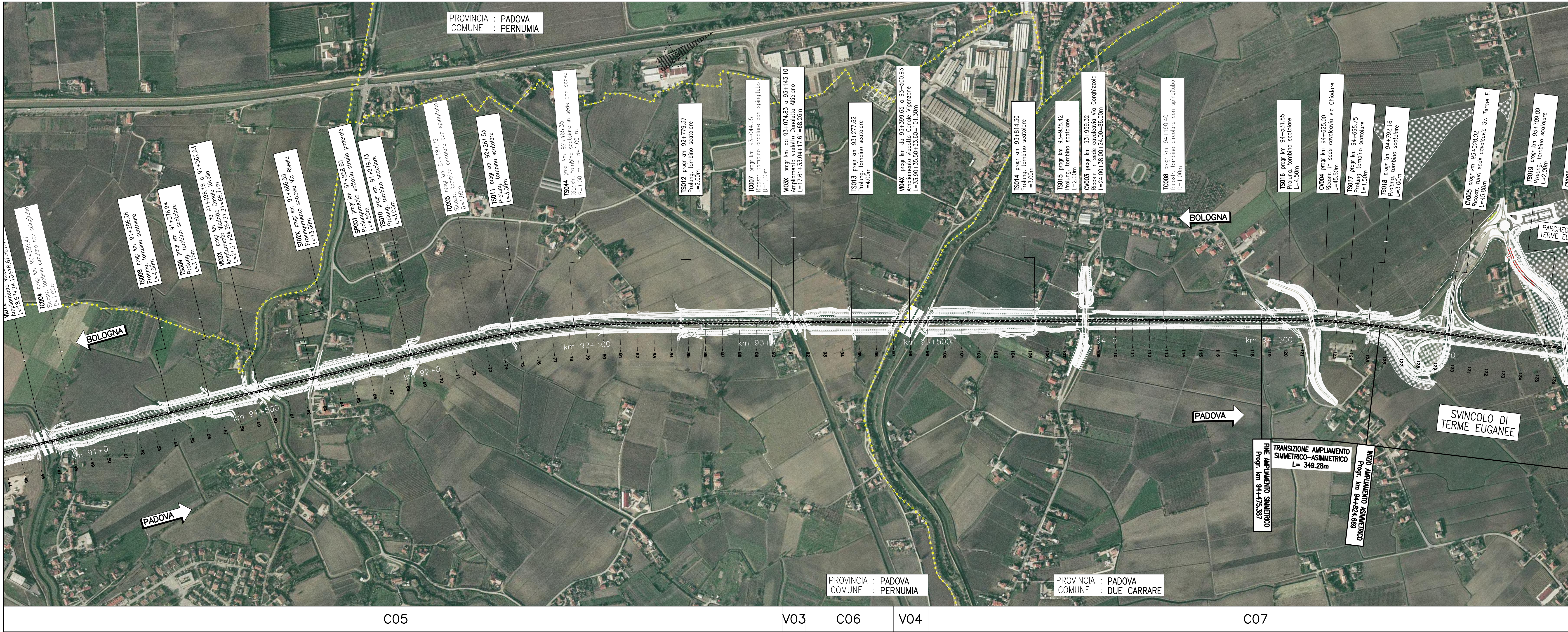
QUADRO 2 – PLANIMETRIA DI PROGETTO SU ORTOFOTO dal km 91+500 al km 94+500 – 1:5.000
