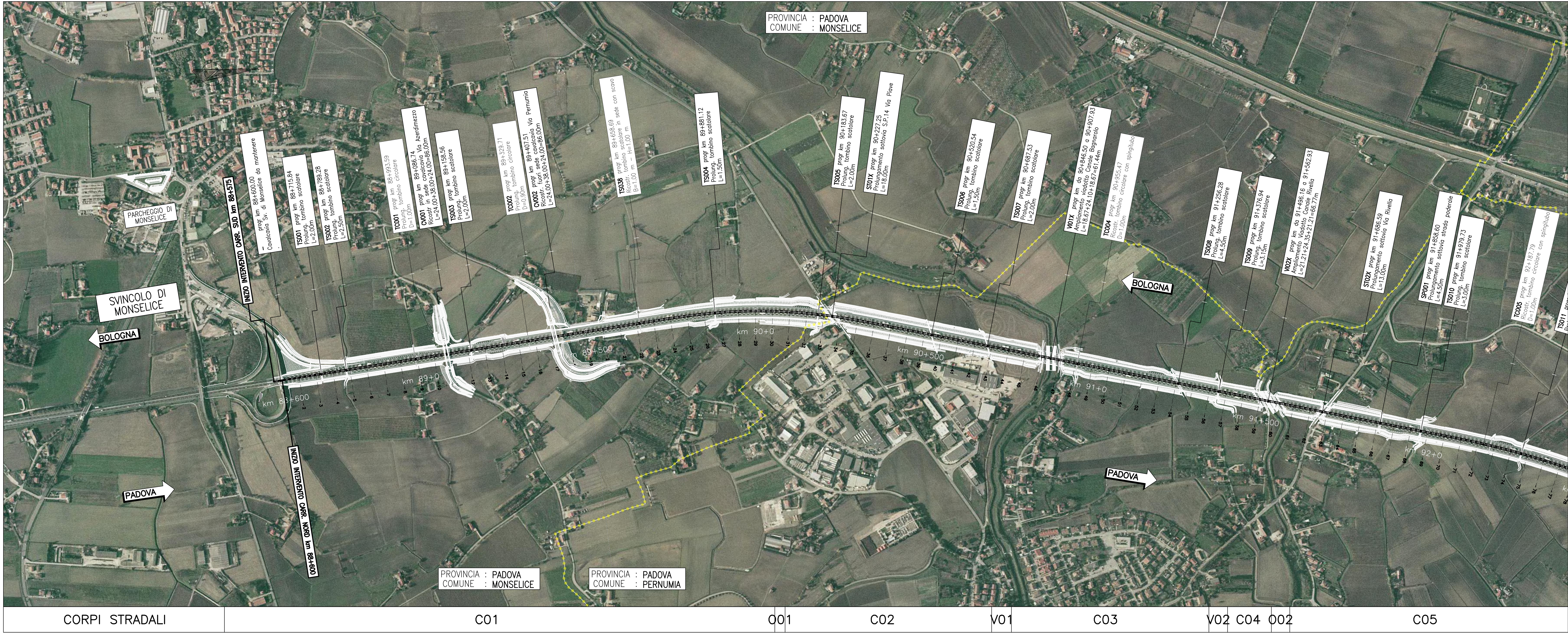
QUADRO 1 – PLANIMETRIA DI PROGETTO SU ORTOFOTO dal km 88+575 al km 91+500 – 1:5.000
