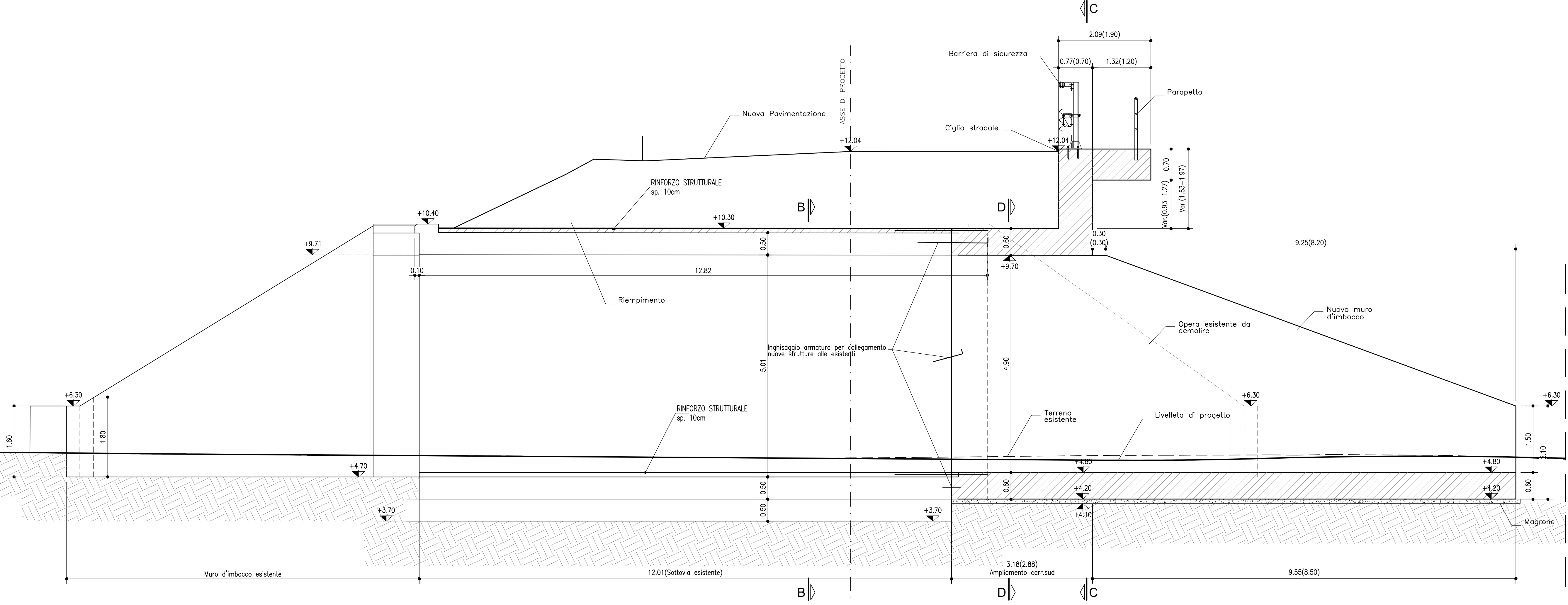
SEZIONE LONGITUDINALE A-A SCALA 1:50
