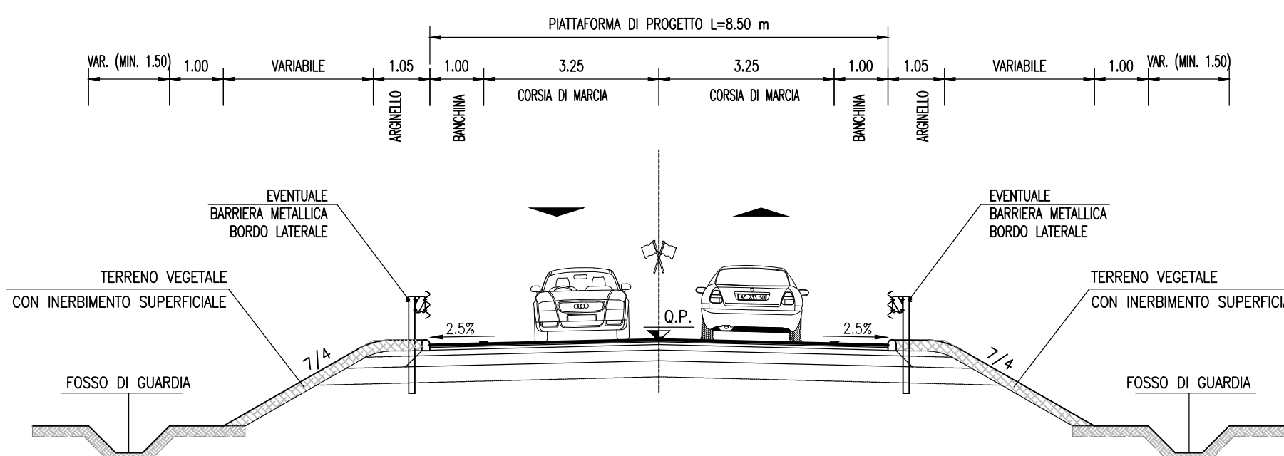
SEZIONE TIPO IN RILEVATO
