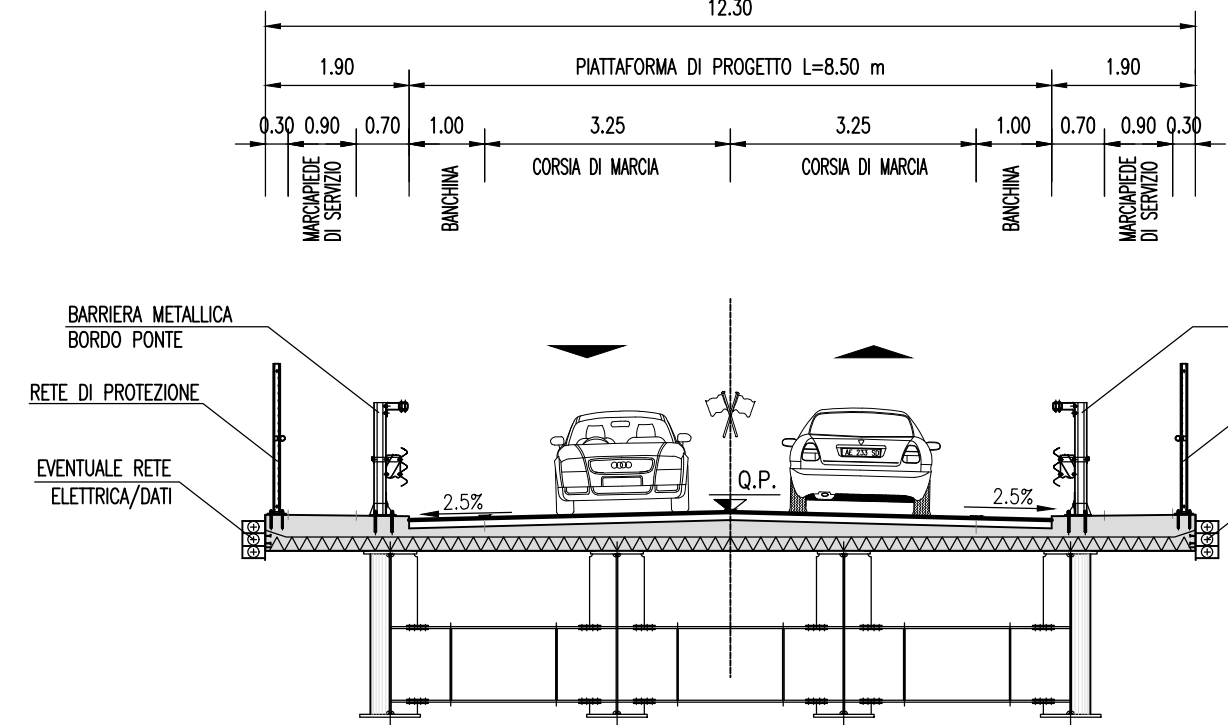
SEZIONE TIPO SU OPERA D'ARTE (CAVALCAVIA)
