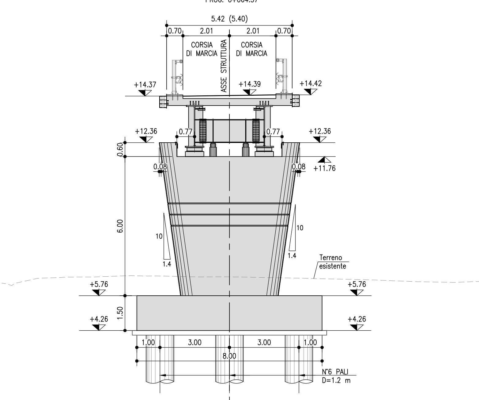
SEZIONE TRASVERSALE SULLA PILA 1 SEZIONE B-B PROG. 0+084.37
