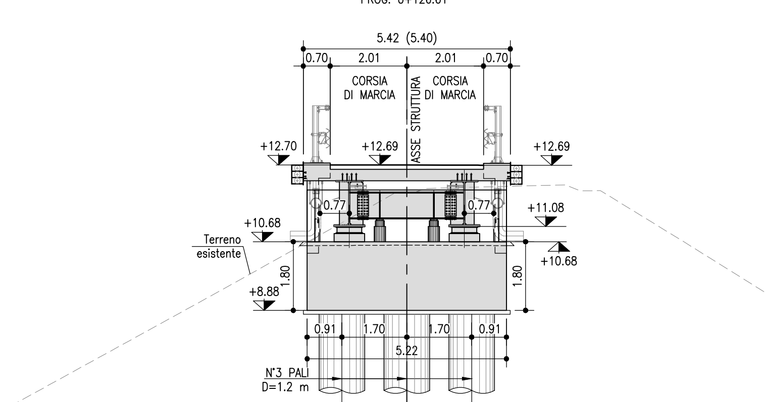
SEZIONE TRASVERSALE SULLA SPALLA B SEZIONE D-D PROG. 0+126.61
