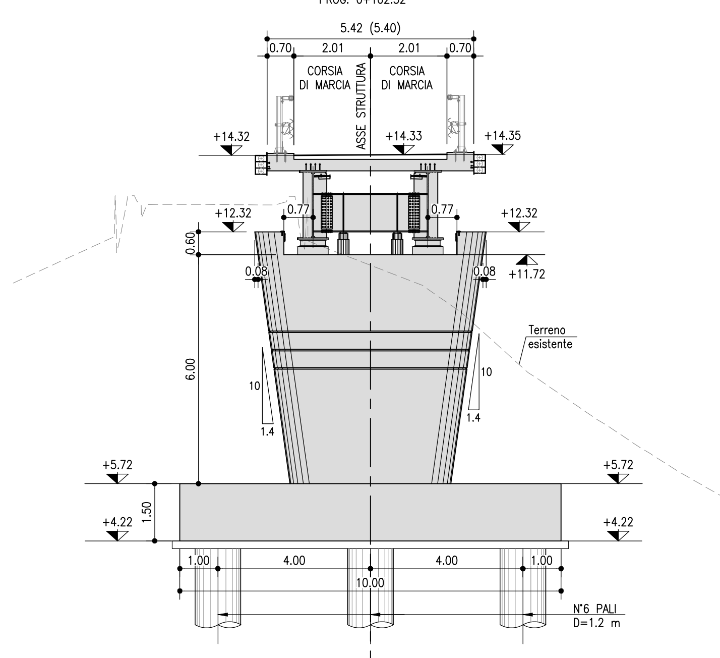
SEZIONE TRASVERSALE SULLA PILA 2 SEZIONE C-C PROG. 0+102.52
