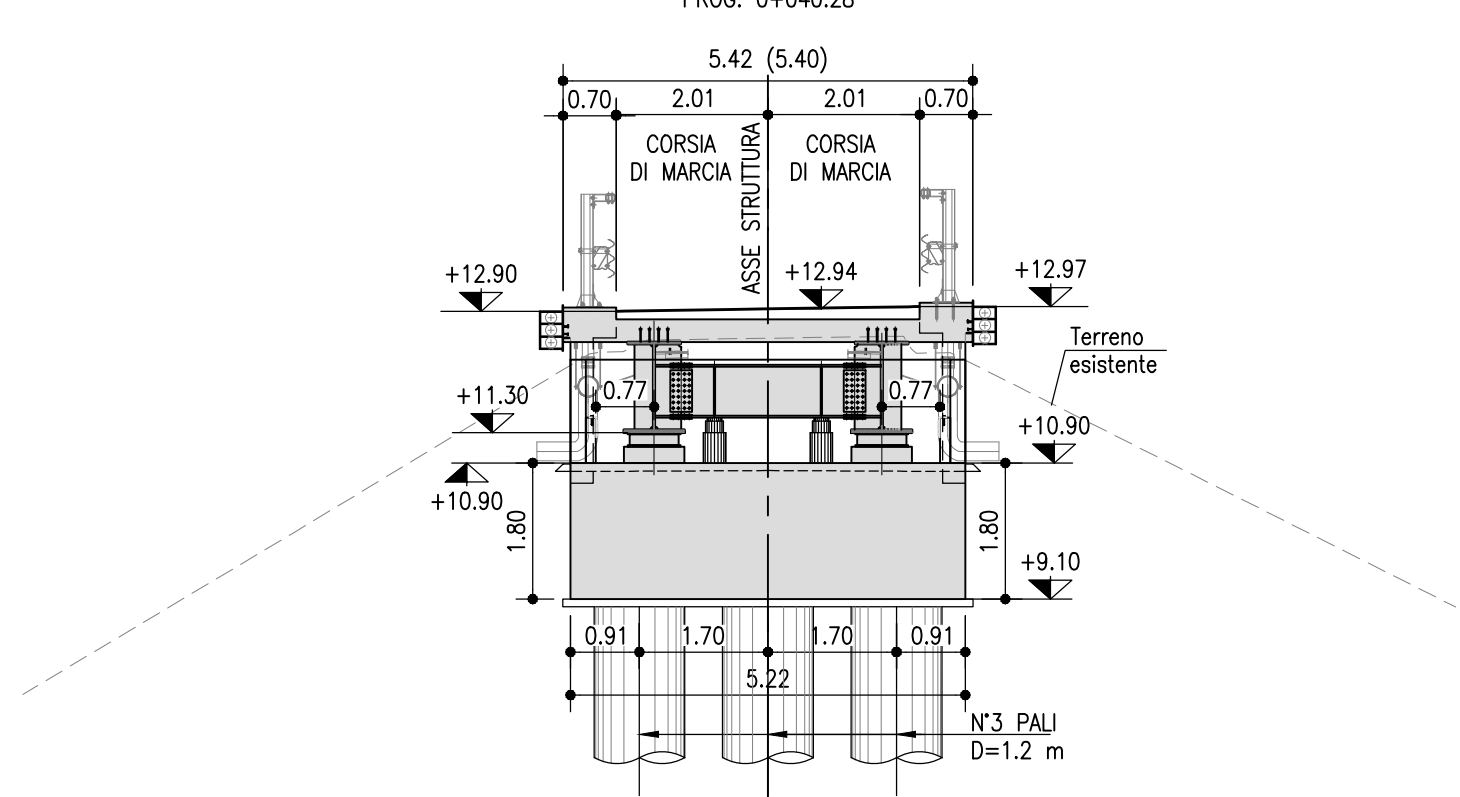
SEZIONE TRASVERSALE SULLA SPALLA A SEZIONE A-A PROG. 0+040.28
