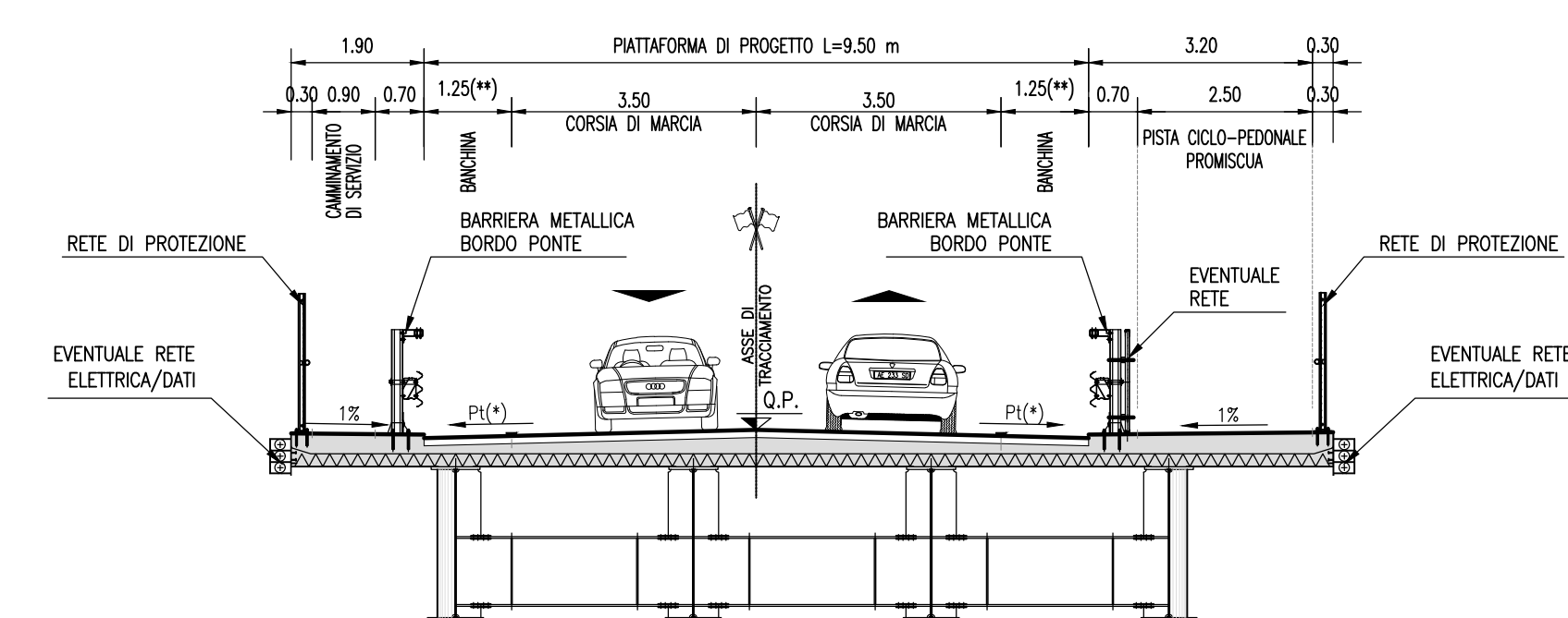
SEZIONE TIPO SU OPERA D'ARTE (CAVALCAVIA)
