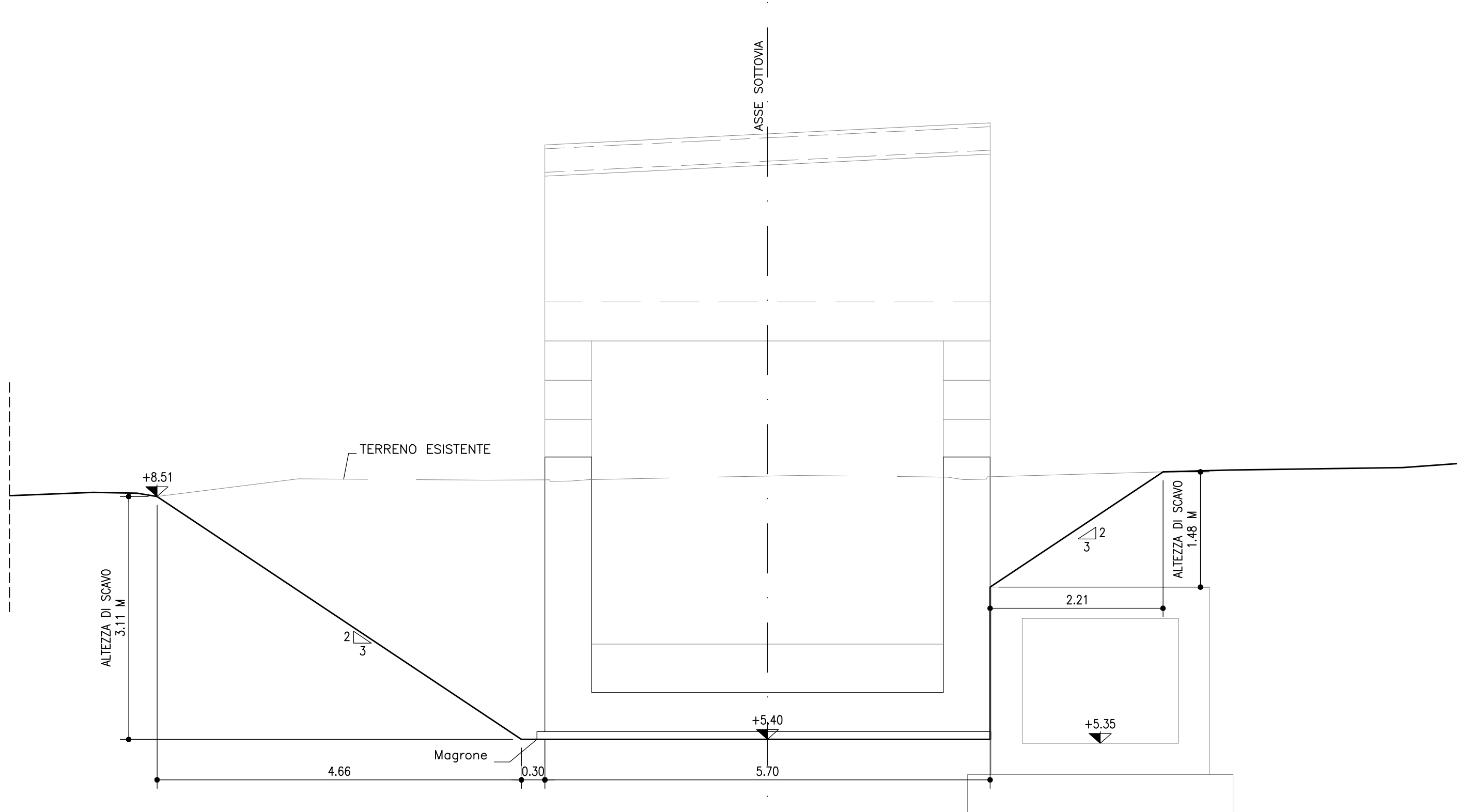
SEZIONE E-E SCALA 1:50
