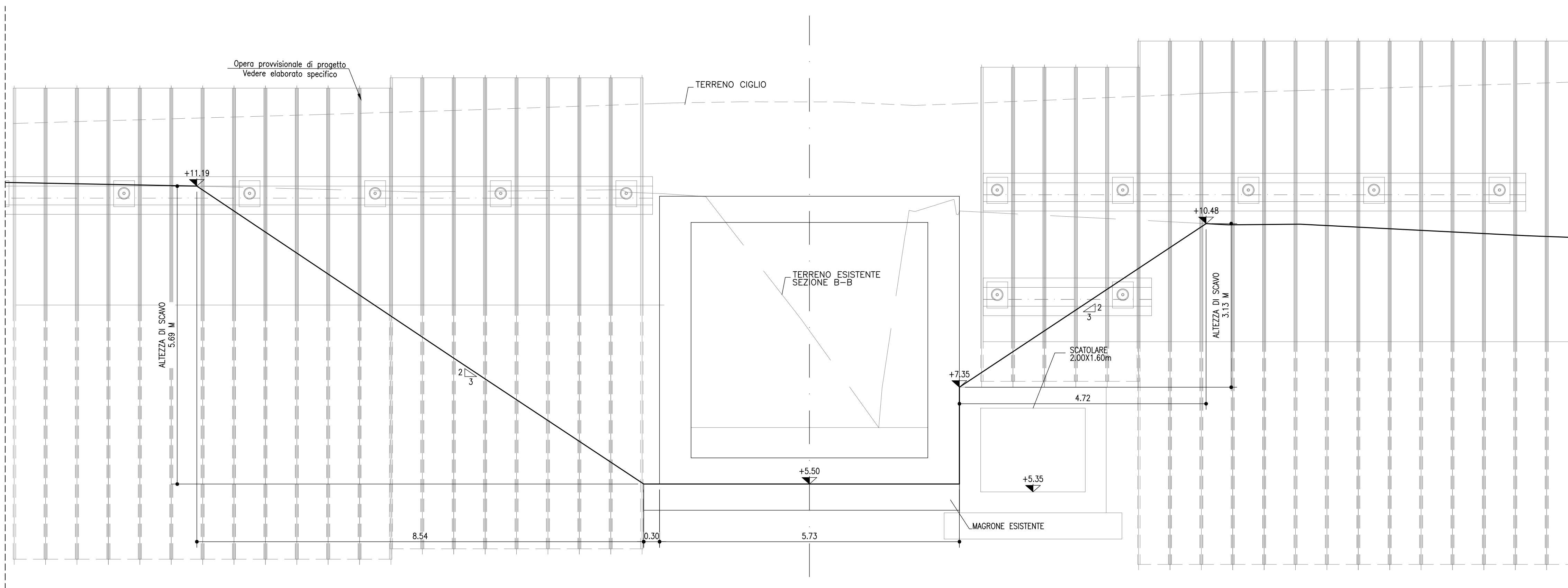
SEZIONE B-B SCALA 1:50
