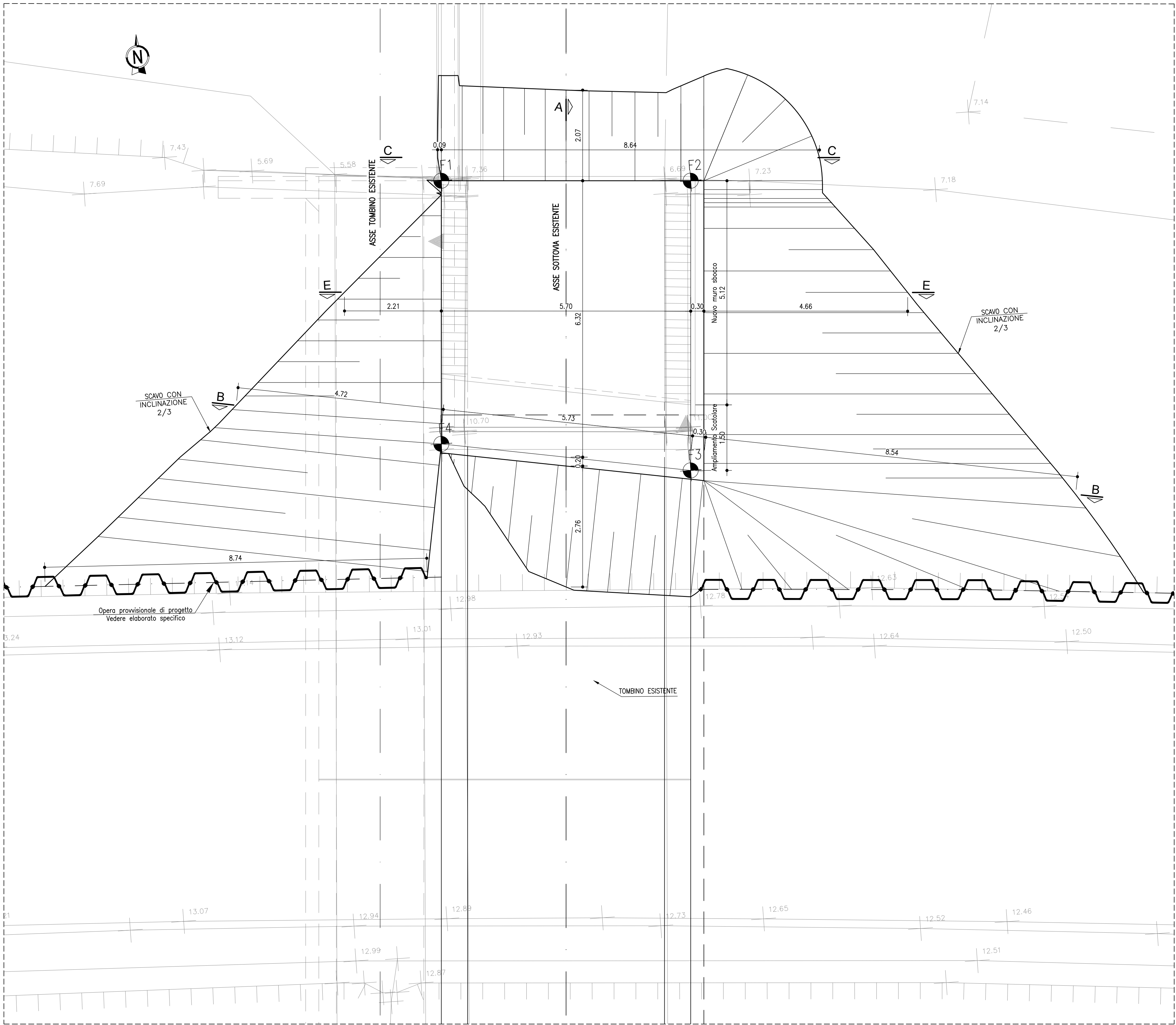
PIANTA GENERALE SCALA 1:50
