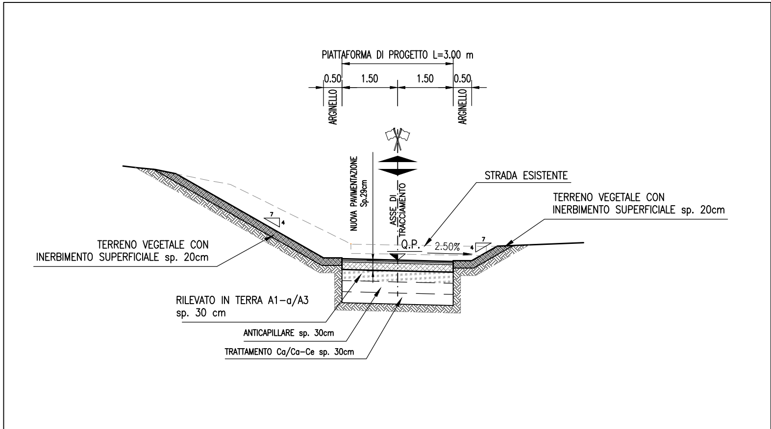
PARTICOLARE PAVIMENTAZIONE scala 1:20
