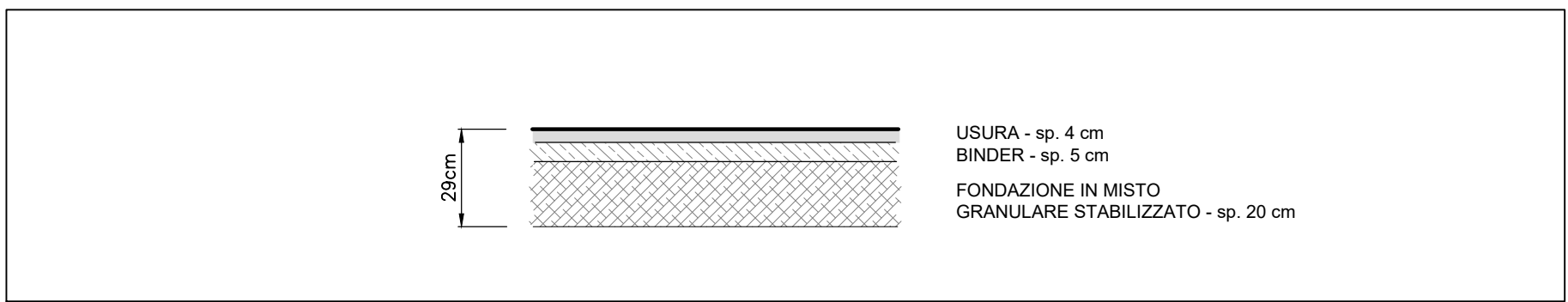
PARTICOLARE PAVIMENTAZIONE scala 1:20
