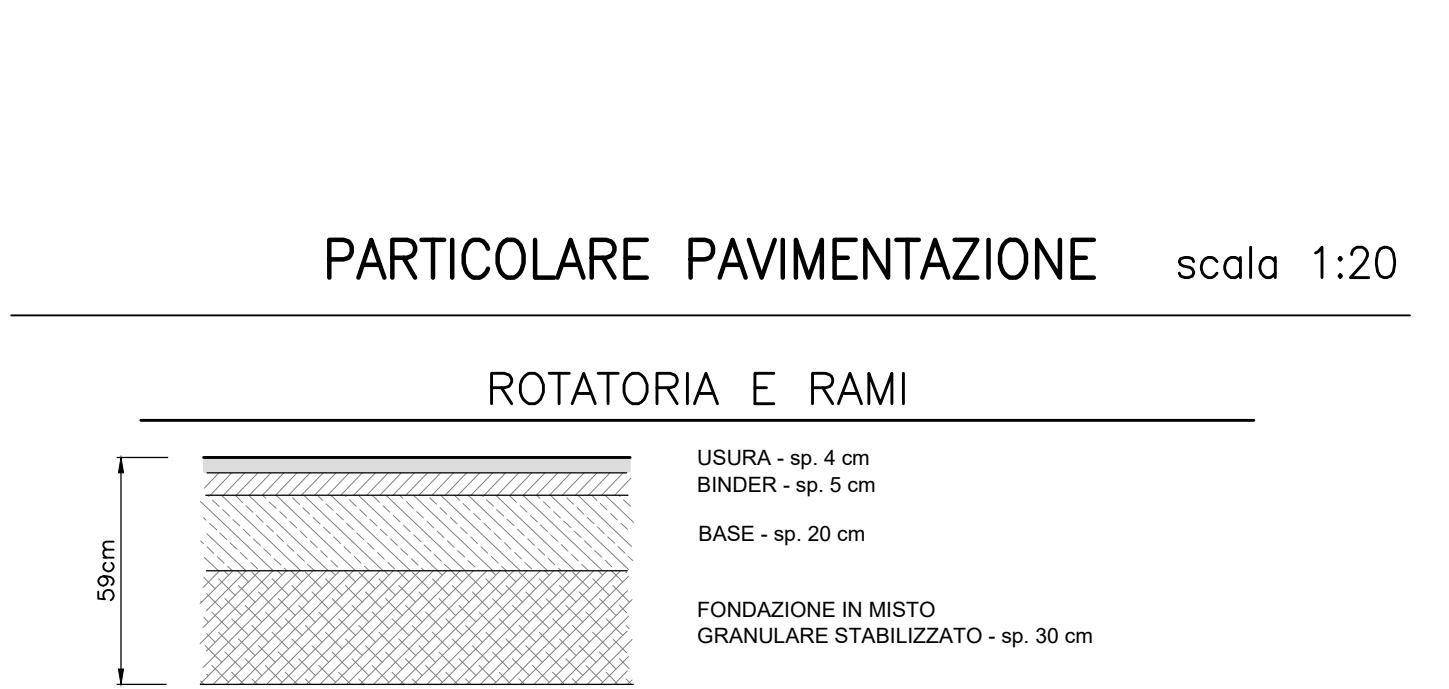
ROTATORIA E RAMI
