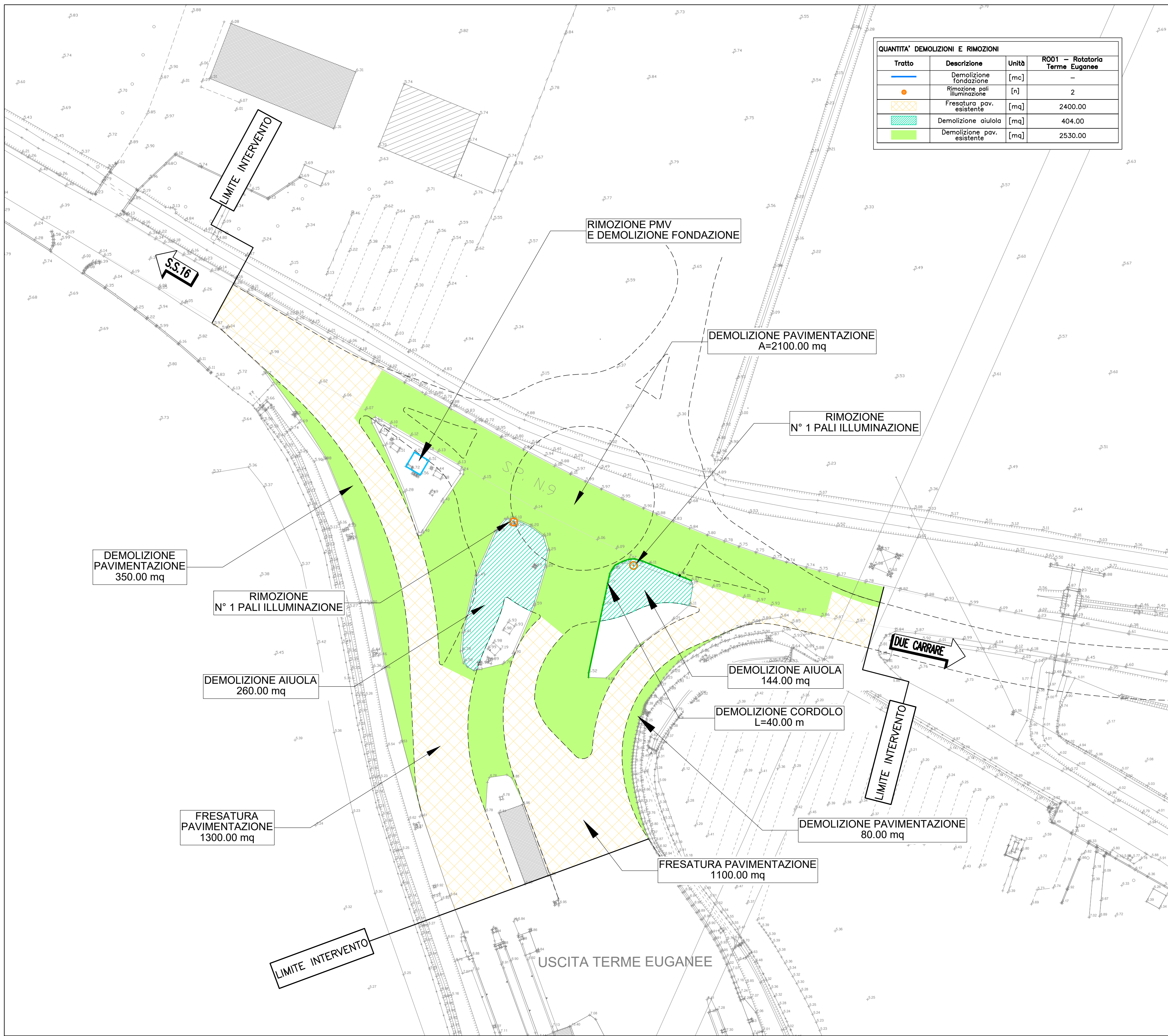
PLANIMETRIA DELLE DEMOLIZIONI E RIMOZIONI scala 1:500
