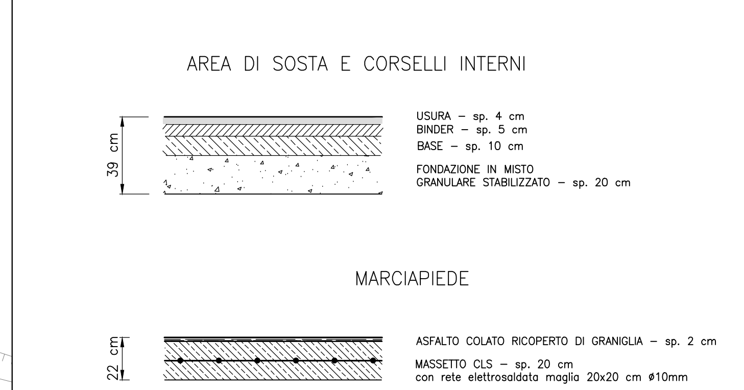
PARTICOLARI PAVIMENTAZIONI
