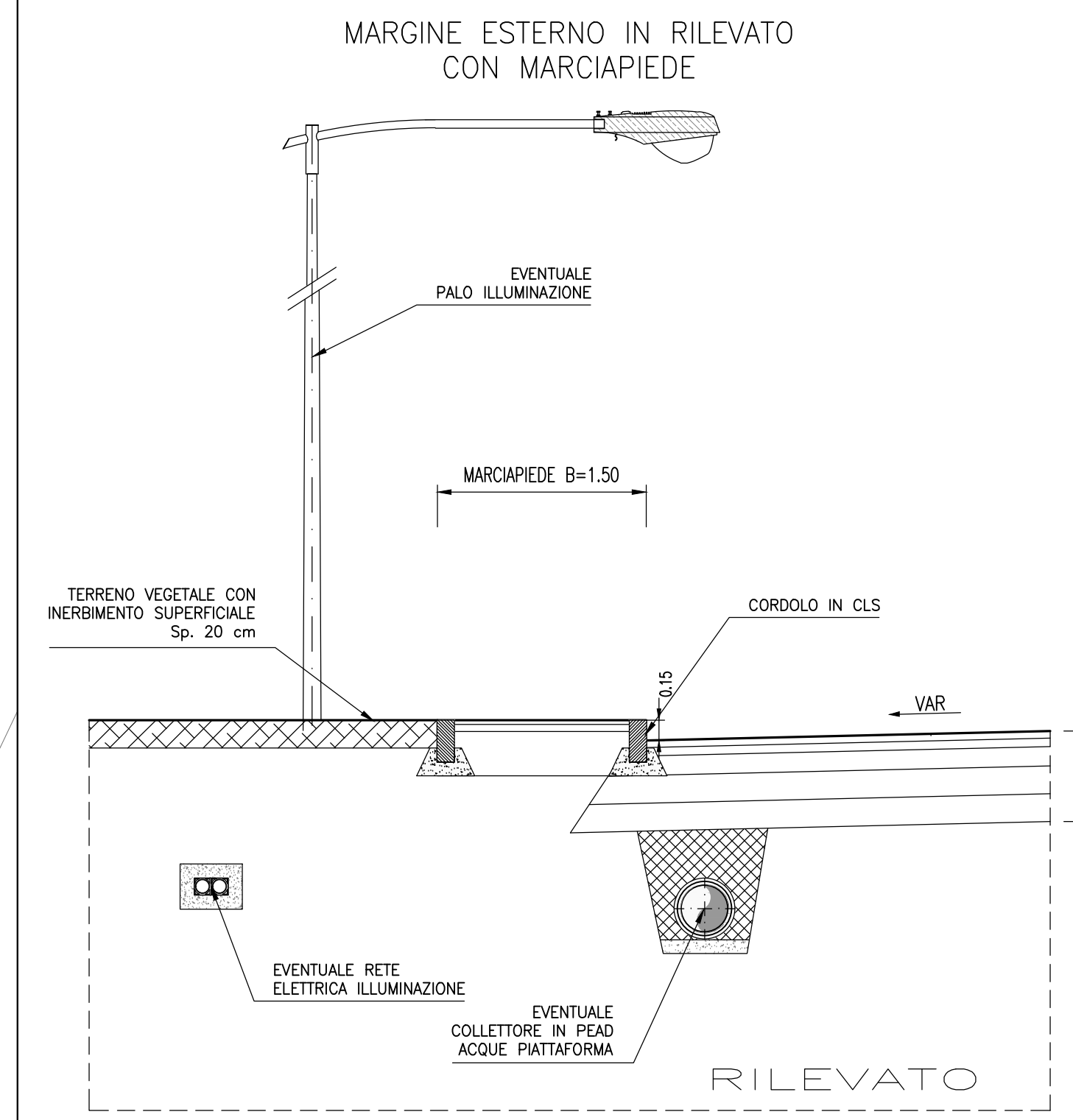
PARTICOLARI PAVIMENTAZIONI
