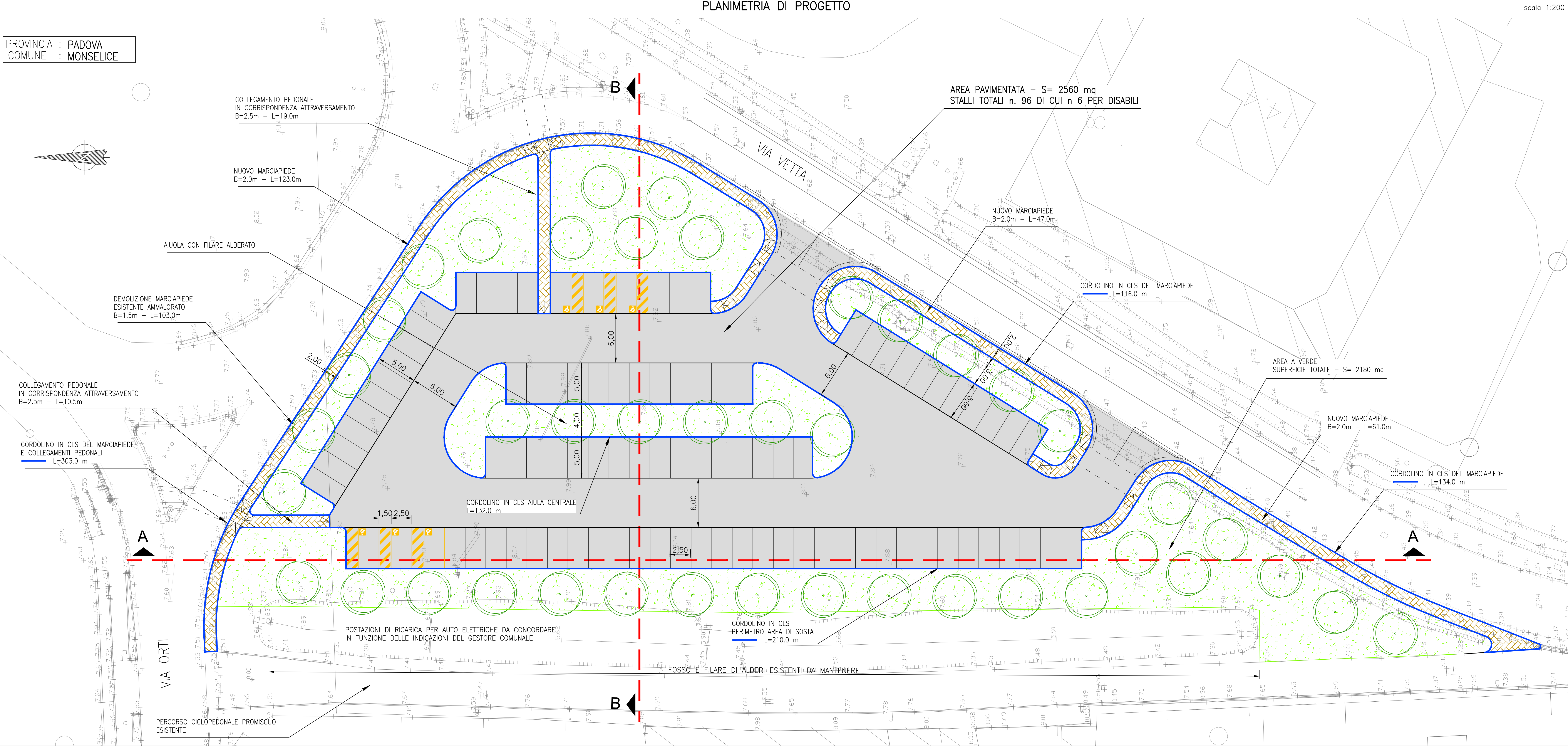
SEZIONI CARATTERISTICA A-A
