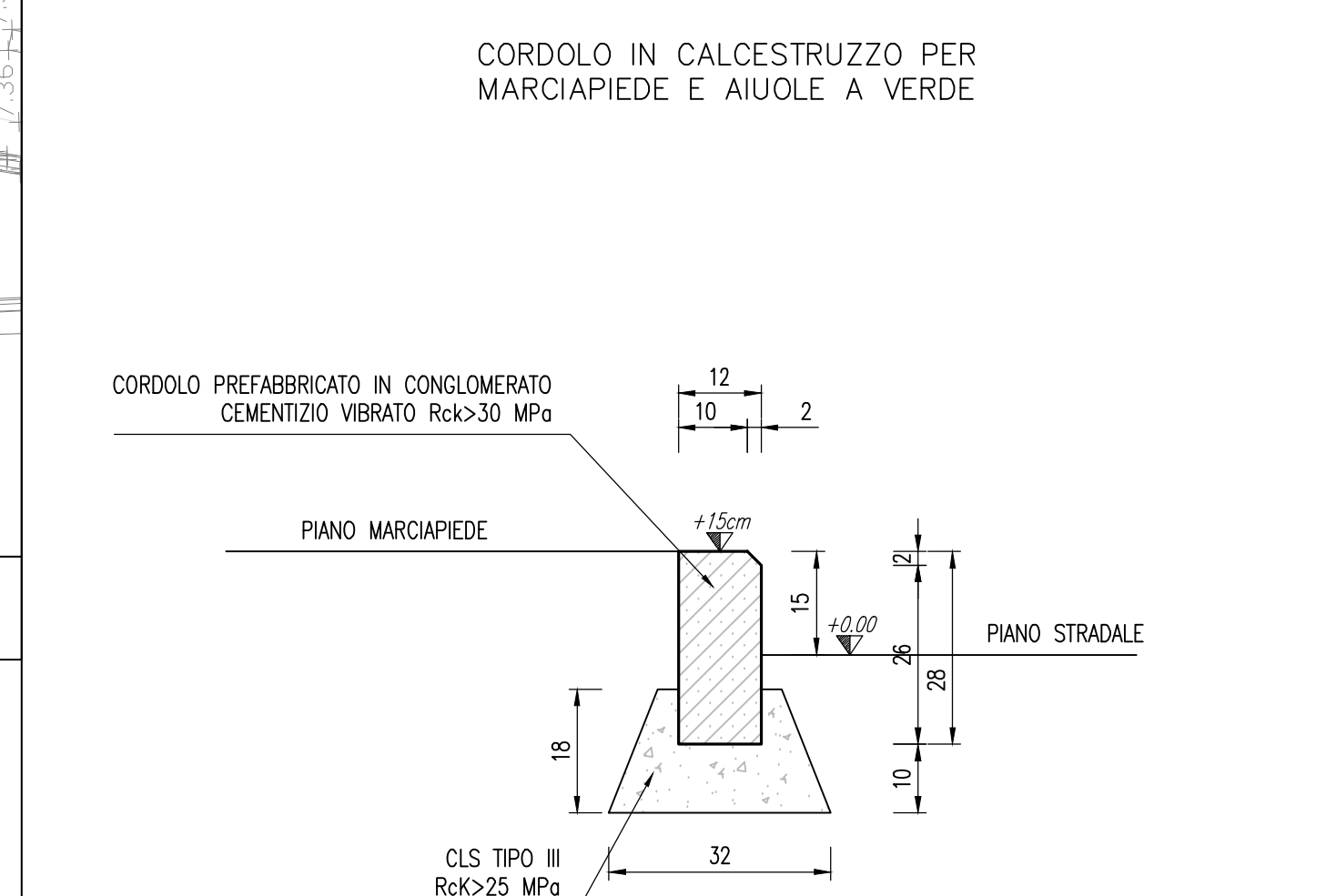
PARTICOLARI CORDOLI
